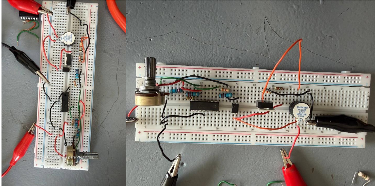
Imagen 2 y 3. Montaje físico del sistema en protoboard
